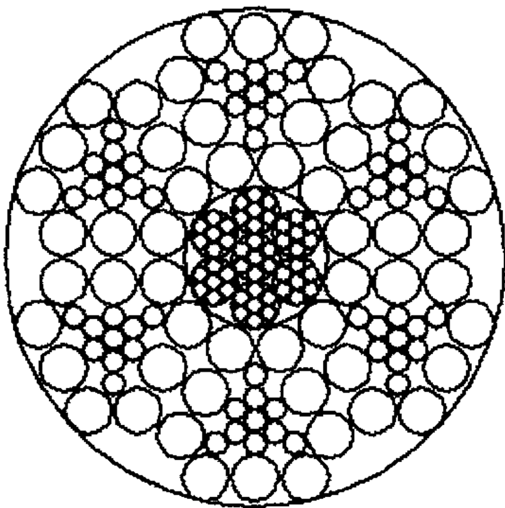
6V×19+IWR
