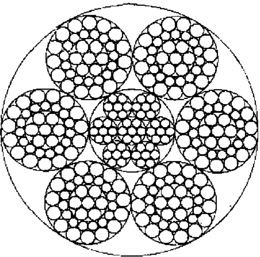
6×37S+IWR
