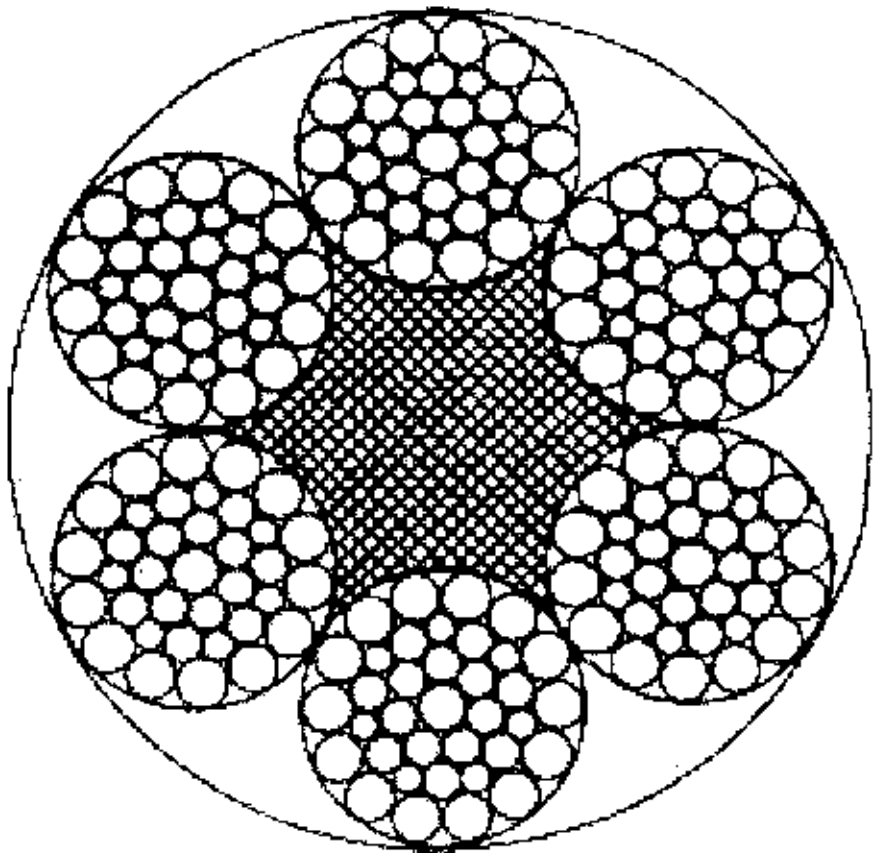
6×36WS+FC
