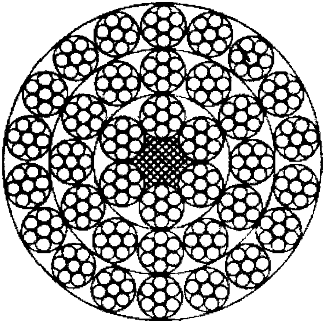
36×7+FC
