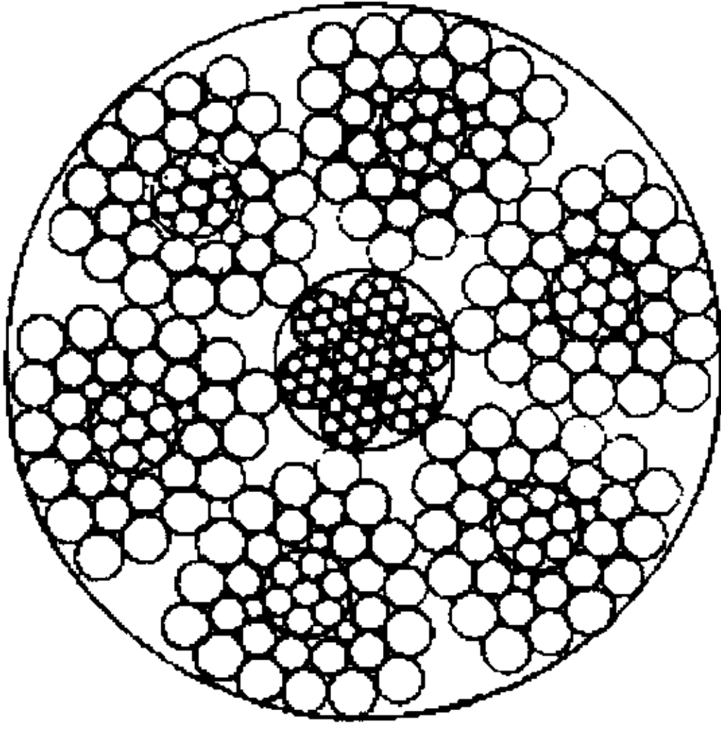
6V×37S+IWR
