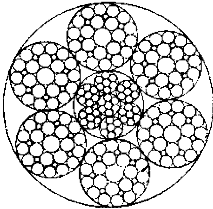
6×29Fi+IWR
