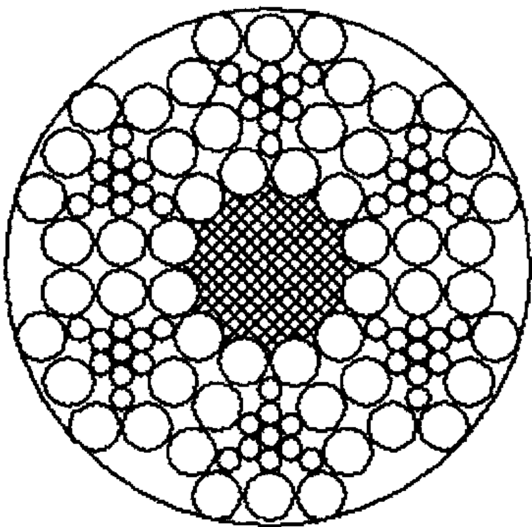
6V×19+FC
