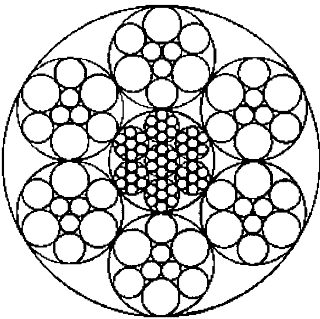
6×9W+IWR
