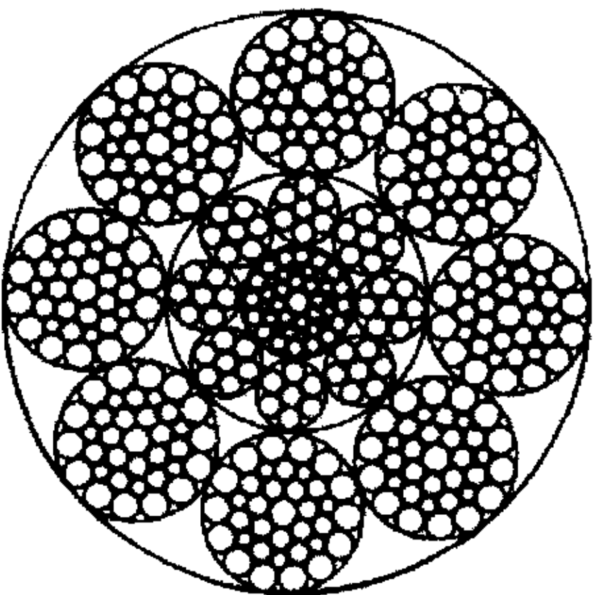
8×36WS+IWR
