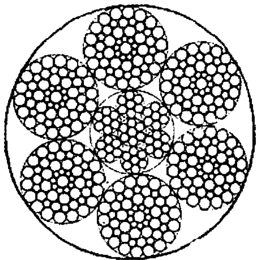
6×55SWS+IWR
