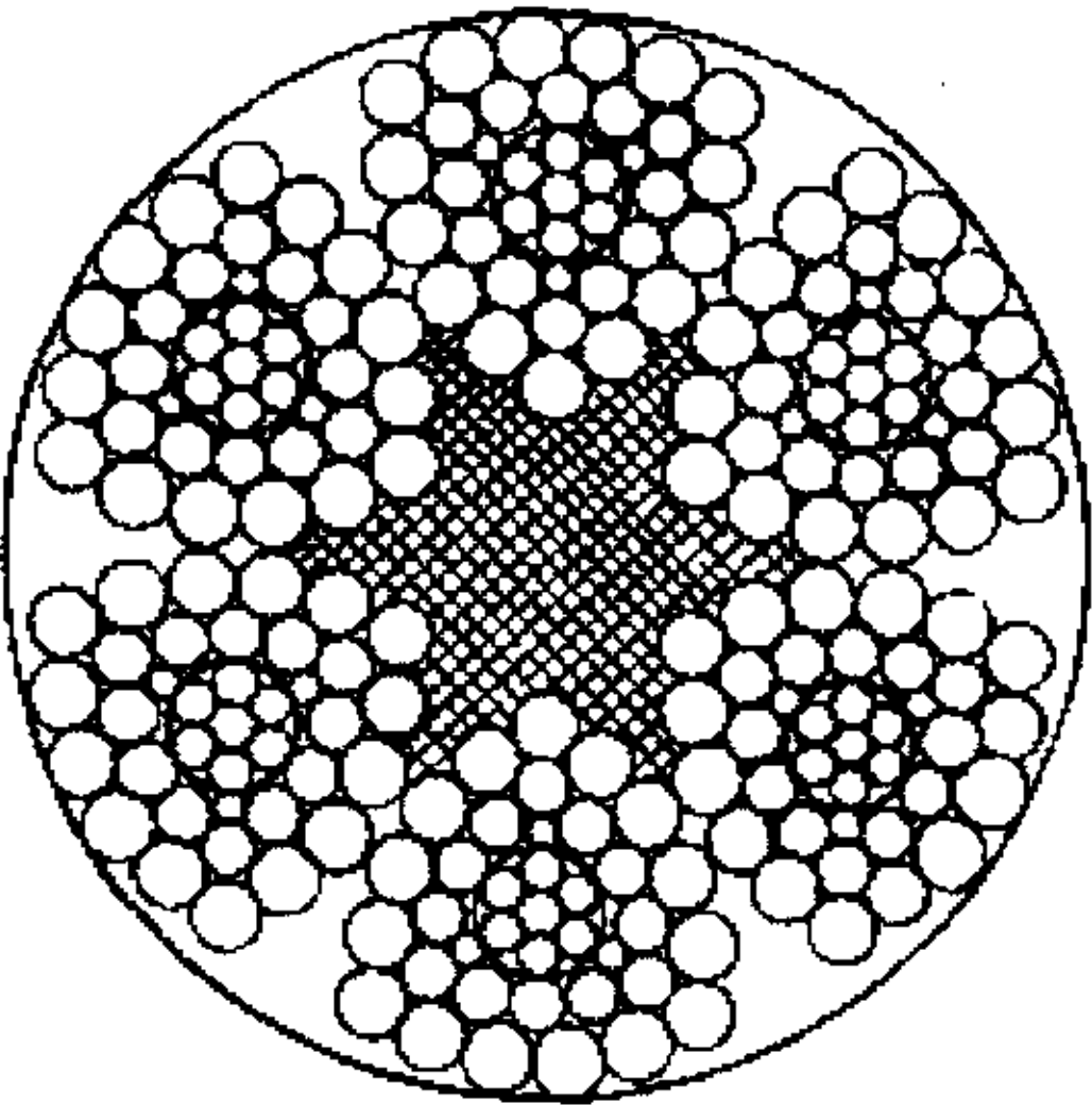
6V×37S+FC
