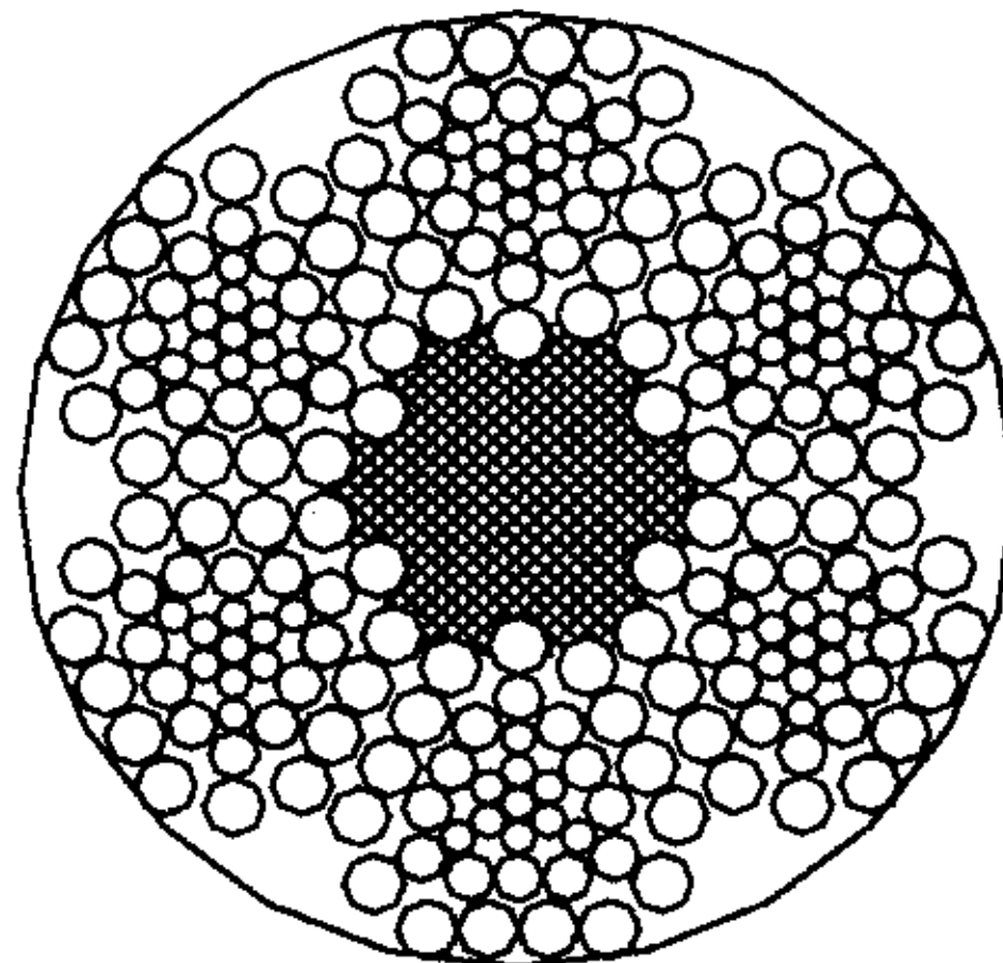
6V×37+FC
