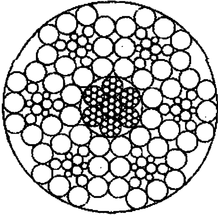
6V×18+IWR
