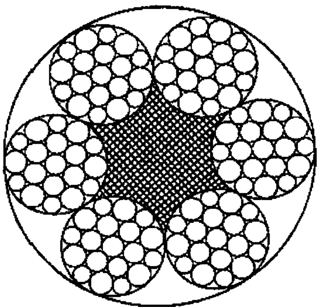
6×19W+FC
