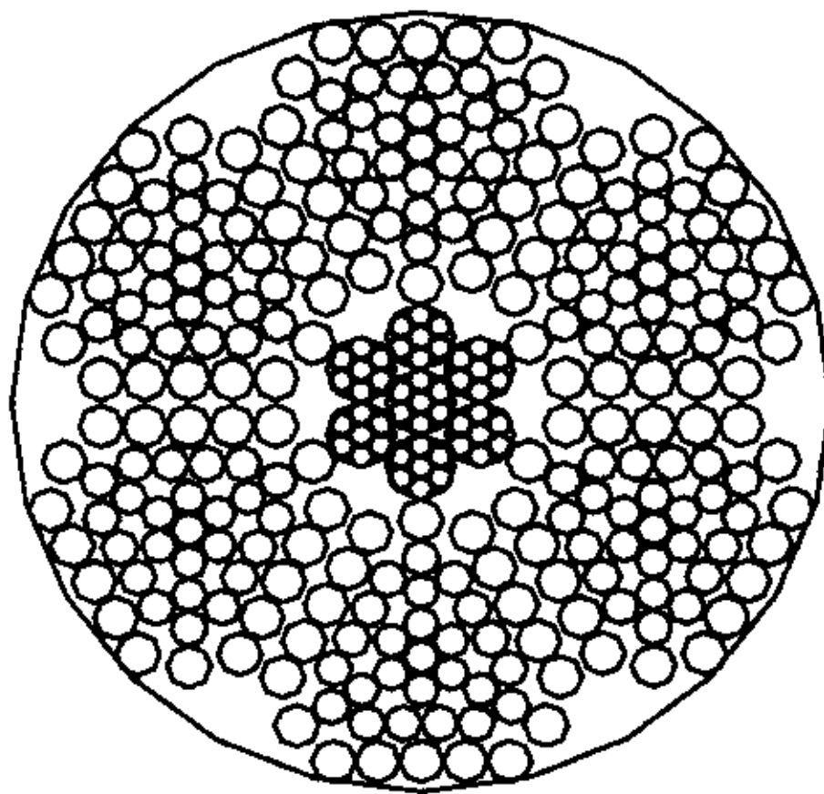
6V×43+IWR
