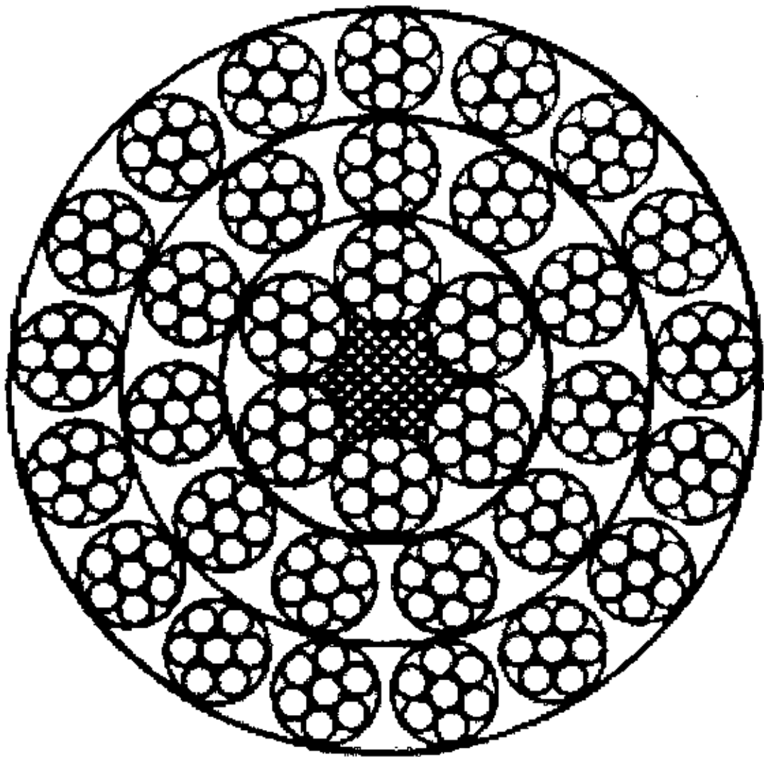
34×7+FC
