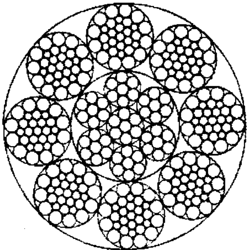
8×31WS+IWR
