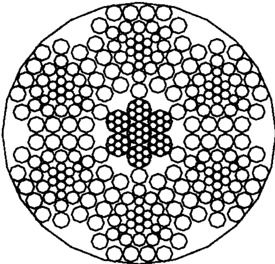
6V×37+IWR
