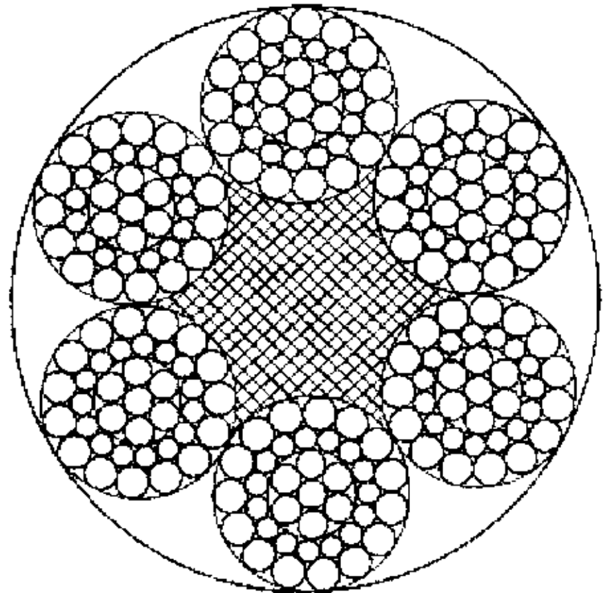
6×37S+FC
