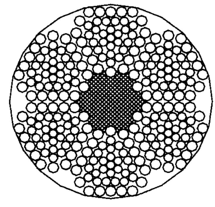
6V×43+FC
