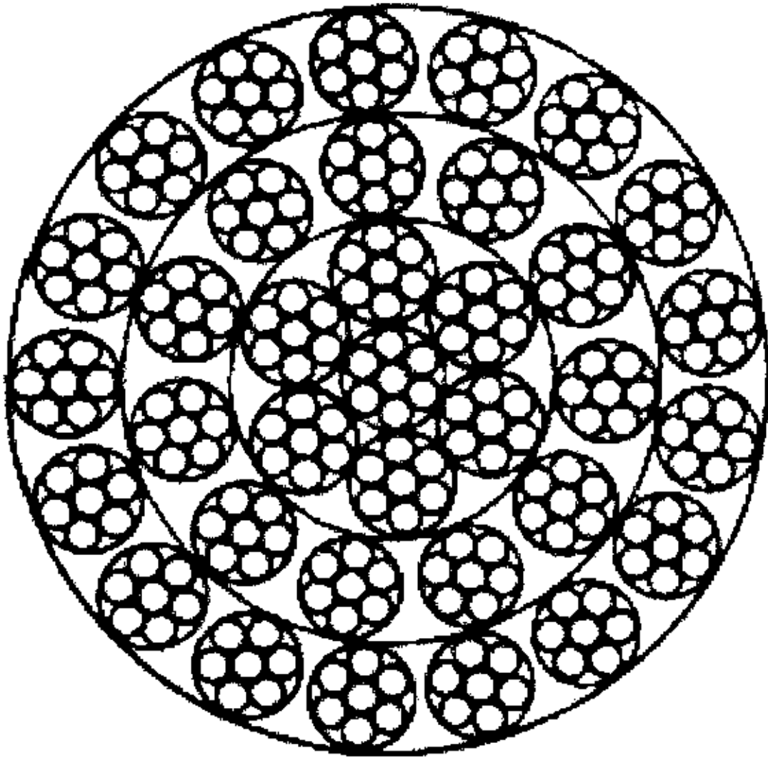
34×7+IWS
