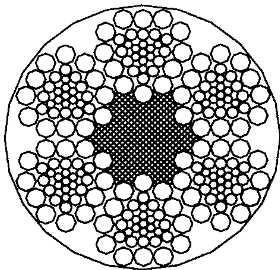
6V×34+FC
