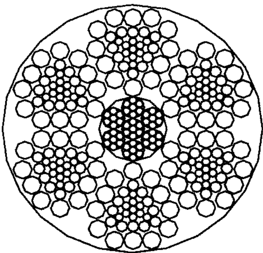
6V×34+IWR
